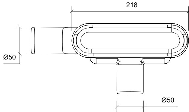
Plan/Plan/Draufsicht
