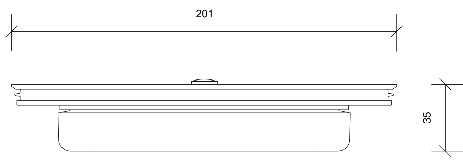
Front Opstalt/Front Elevation/Frontansicht
