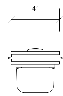
Side Opstalt/Side Elevation/Seitenansicht
