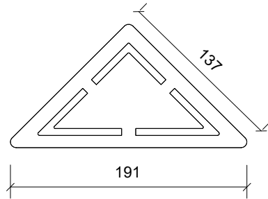
Plan/Plan/Draufsicht
