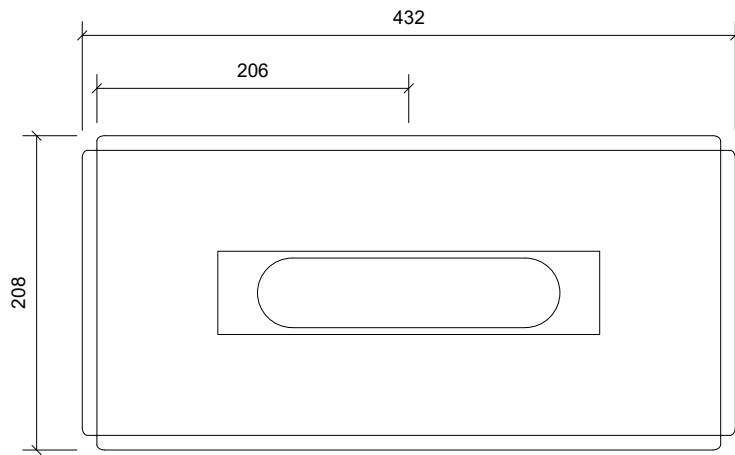
Plan/Plan/Draufsicht
