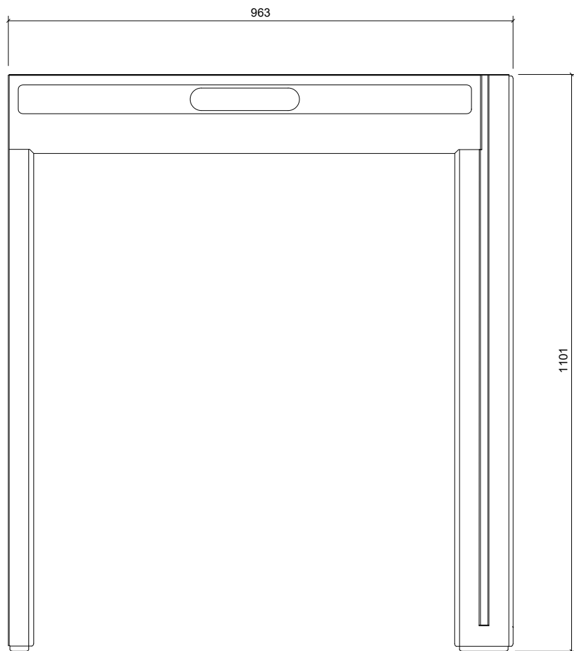
Plan/Plan/Draufsicht
