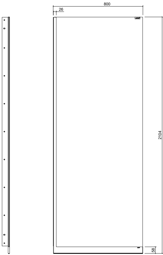
Side Opstalt/Side Elevation/Seitenansicht
