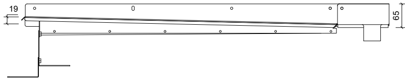
Side Opstalt/Side Elevation/Seitenansicht
