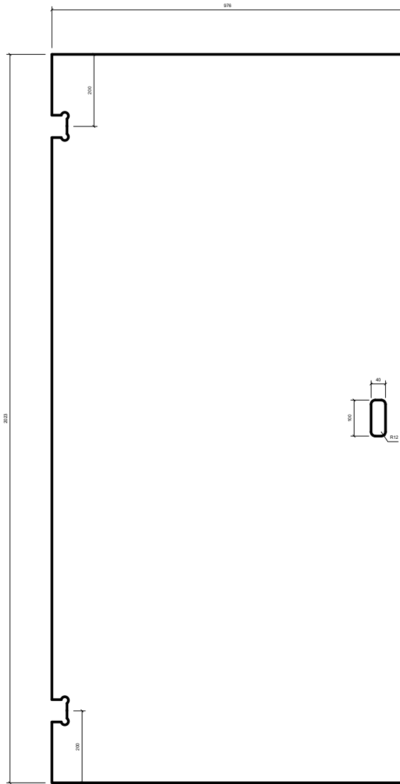
Front Opstalt/Front Elevation/Frontansicht
