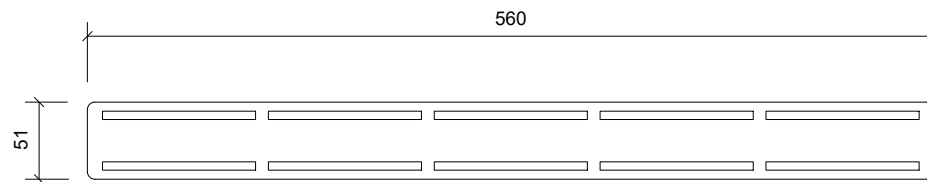
Plan/Plan/Draufsicht
