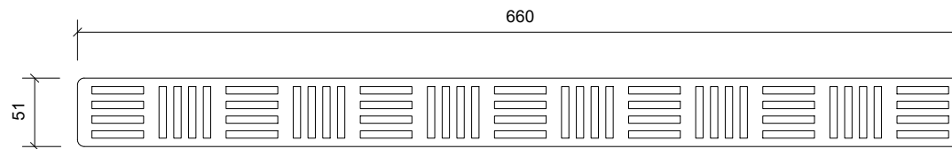
Plan/Plan/Draufsicht
