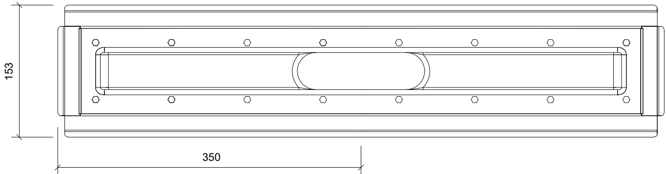
Plan/Plan/Draufsicht
