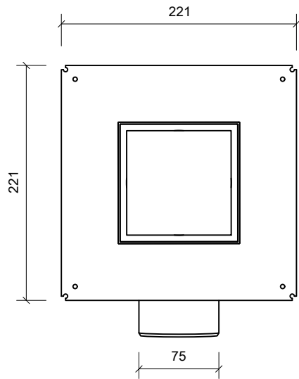
Plan/Plan/Draufsicht
