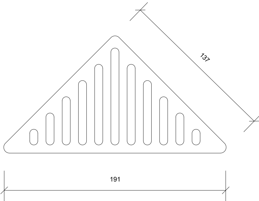
Plan/Plan/Draufsicht
