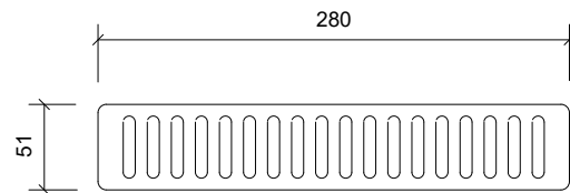
Plan/Plan/Draufsicht
