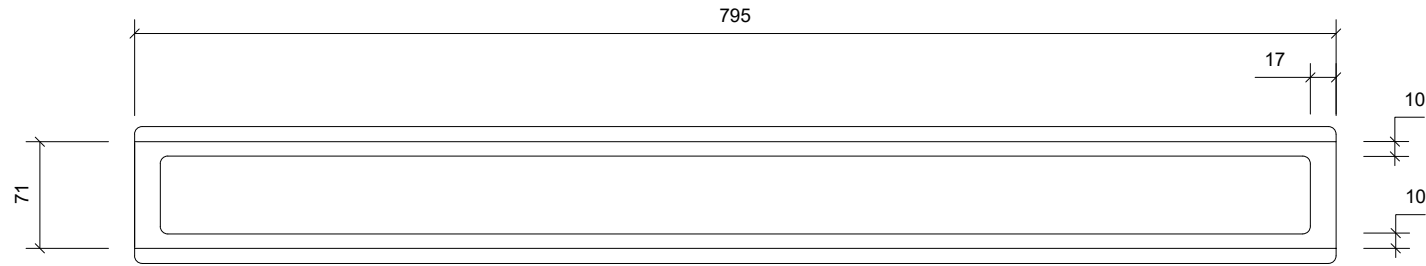
Plan/Plan/Draufsicht
