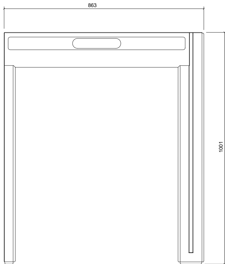
Plan/Plan/Draufsicht
