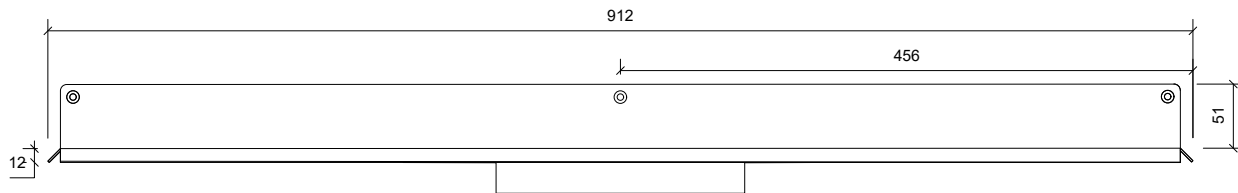
Front Opstalt/Front Elevation/Frontansicht
