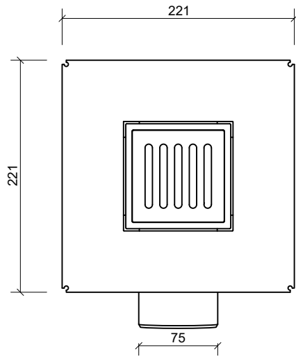
Plan/Plan/Draufsicht
