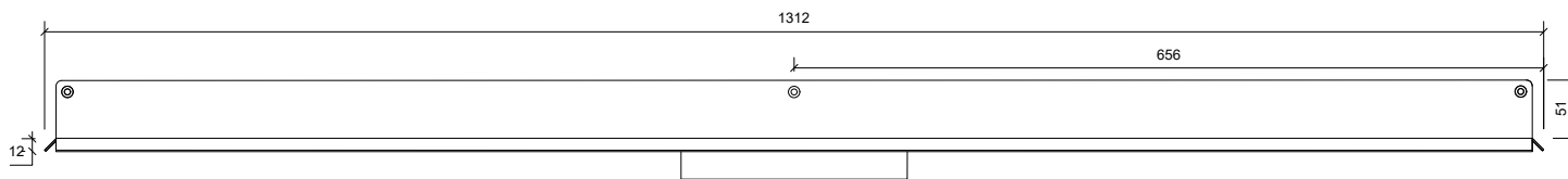
Front Opstal/Front Elevation/Frontansicht
