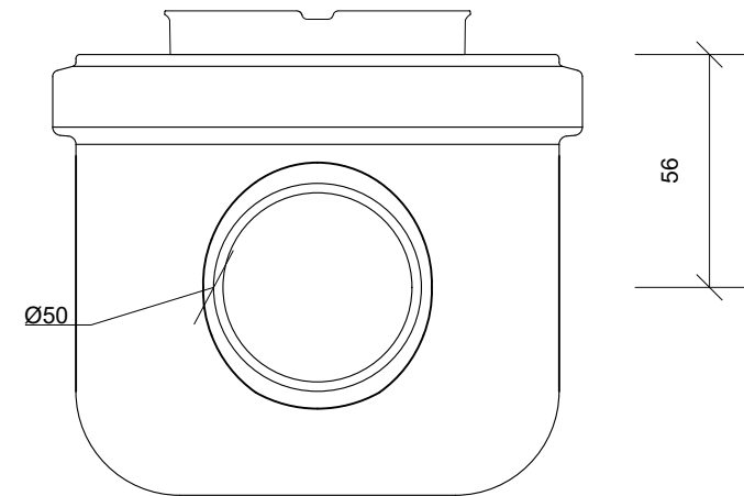
Front Opstalt/Front Elevation/Frontansicht
