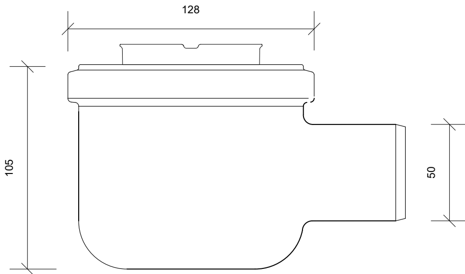
Side Opstalt/Side Elevation/Seitenansicht
