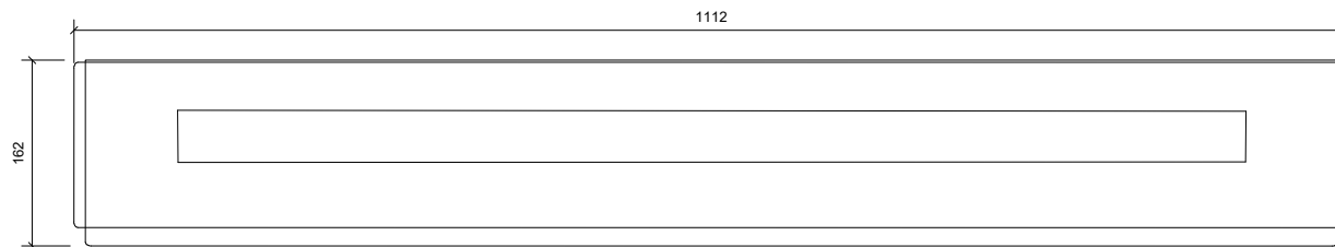
Plan/Plan/Draufsicht
