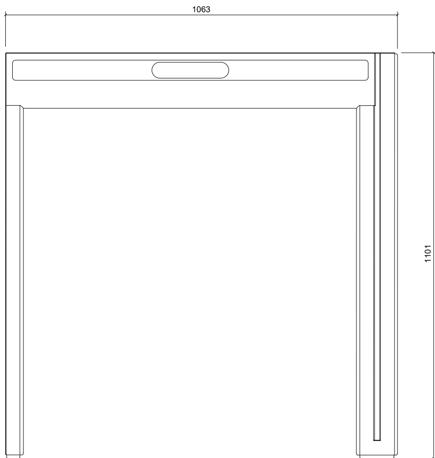
Plan/Plan/Draufsicht
