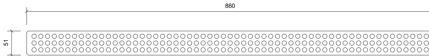
Plan/Plan/Draufsicht
