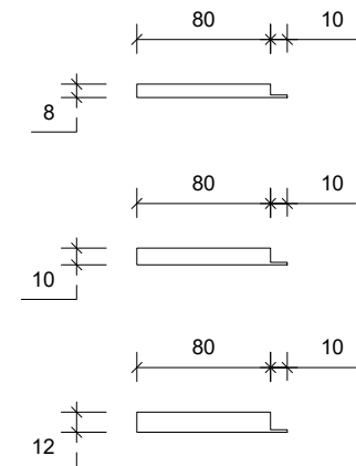
Side Opstalt/Side Elevation/Seitenansicht
