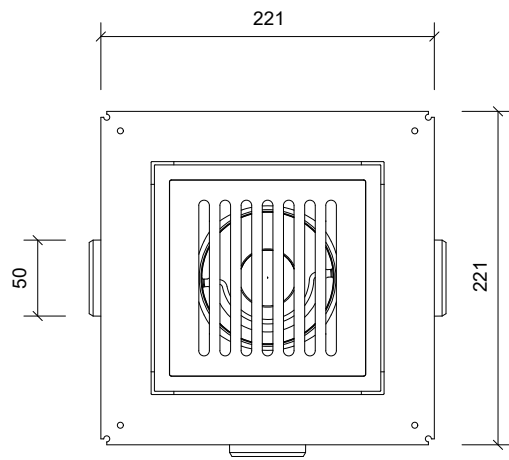
Plan/Plan/Draufsicht
