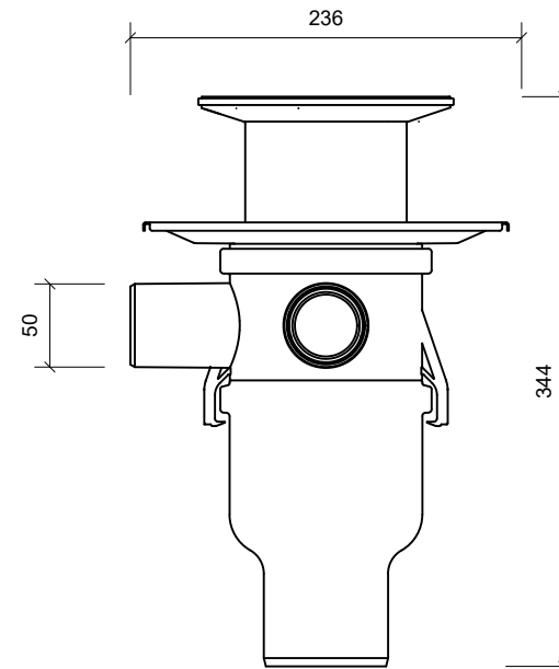
Side Opstalt/Side Elevation/Seitenansicht
