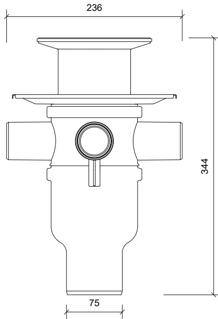
Front Opstalt/Front Elevation/Frontansicht
