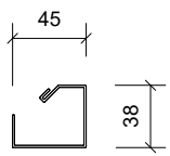
Side Opstalt/Side Elevation/Seitenansicht
