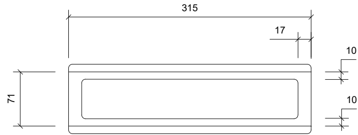
Plan/Plan/Draufsicht
