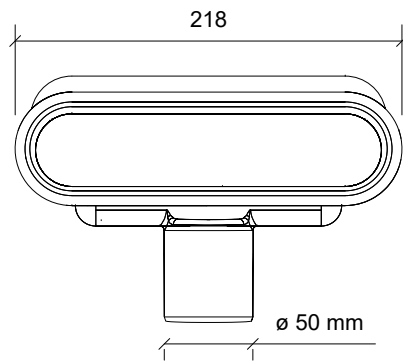
Plan/Plan/Draufsicht
