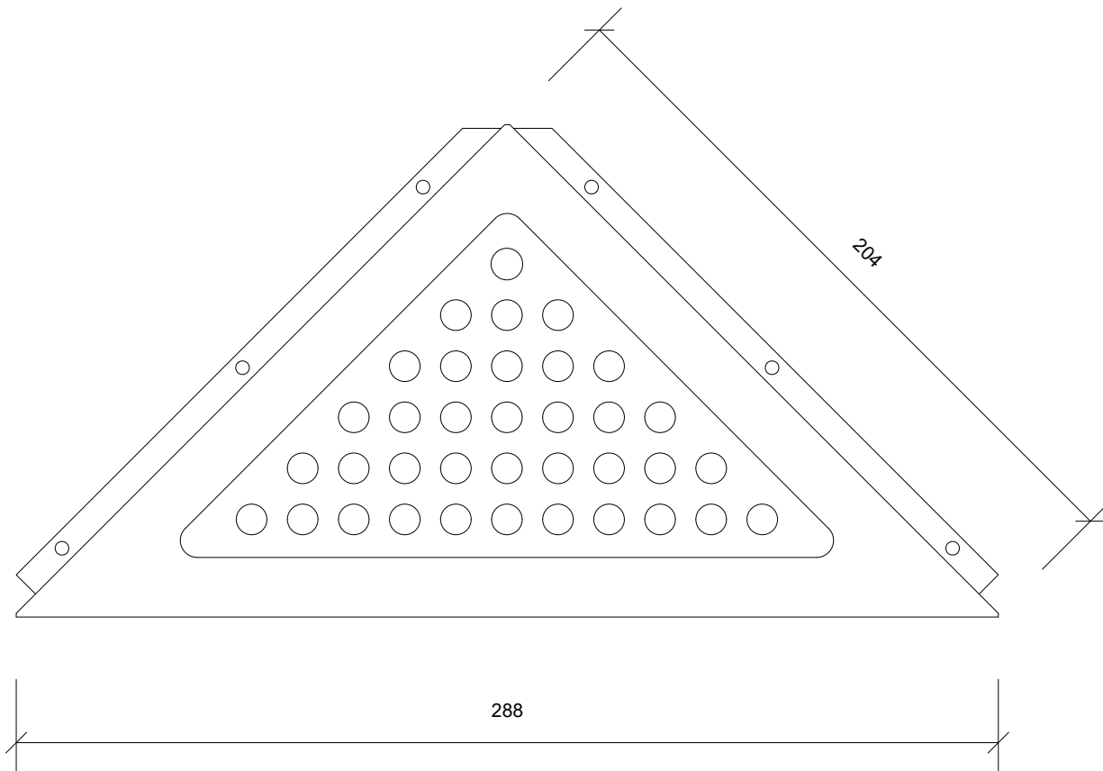
Plan/Plan/Draufsicht
