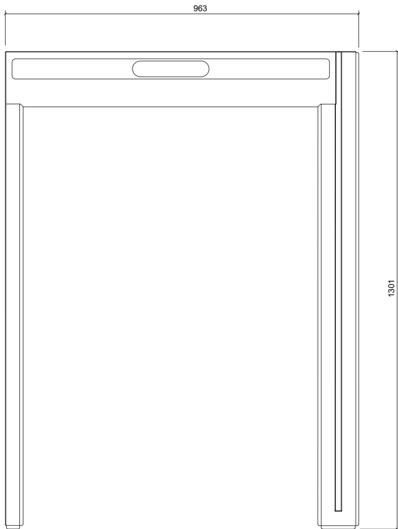
Plan/Plan/Draufsicht
