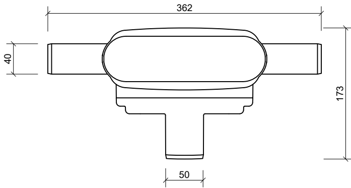
Plan/Plan/Draufsicht
