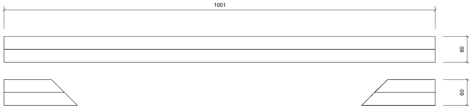
Plan/Plan/Draufsicht
