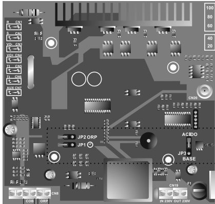
Dosierungpumpe Sicherung (MOD XX - PH) 5x20 T 500 mA/250V
